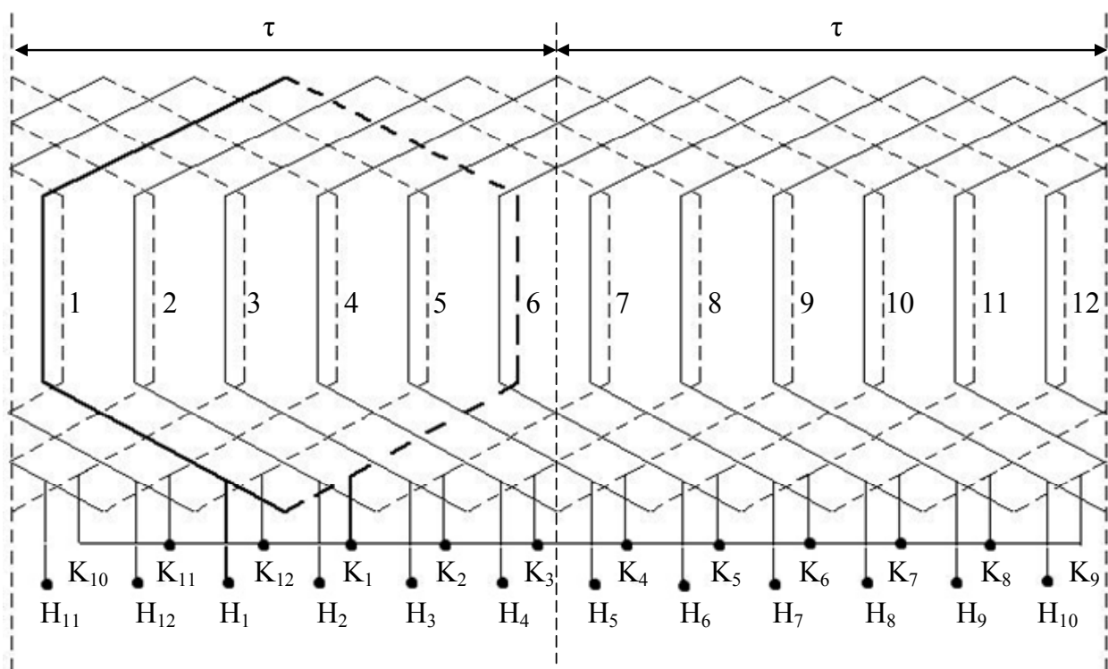
Рис. 1 – 12-фазна обмотка якоря синхронного збудника БСМ
