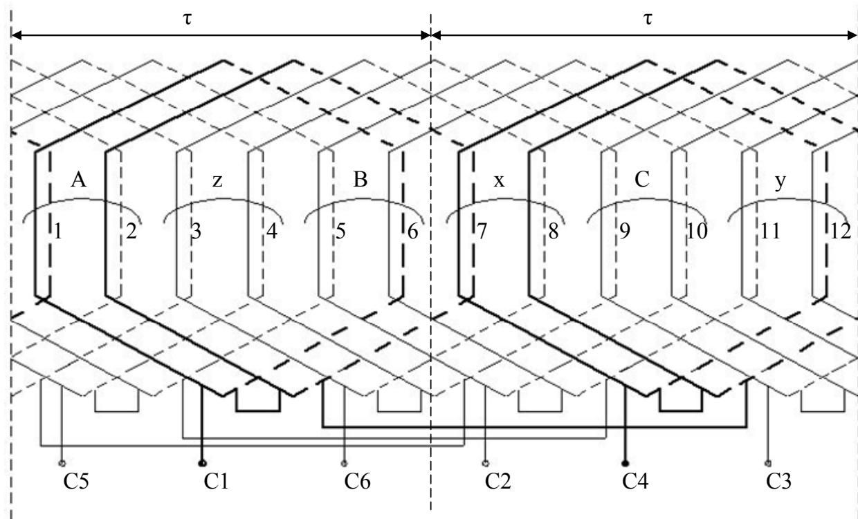
Рис. 2 – 3-фазна обмотка якоря синхронного збудника БСМ
