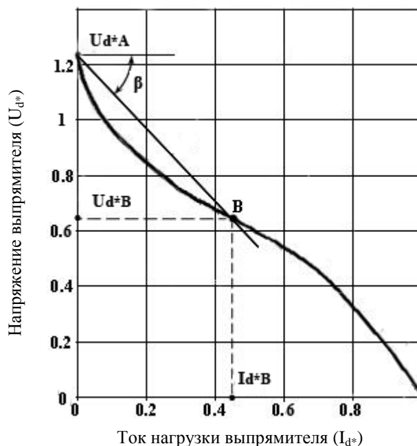
Рисунок 4 – Определение угла наклона внешней характеристики выпрямителя
