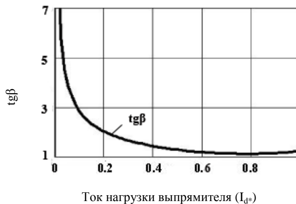
Рисунок 5 – Зависимость \operatorname{tg}\beta от тока I_{d*}
